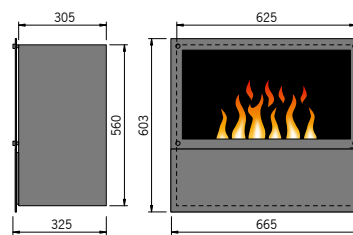
Inside-Front mit 2 Brenner Medium
