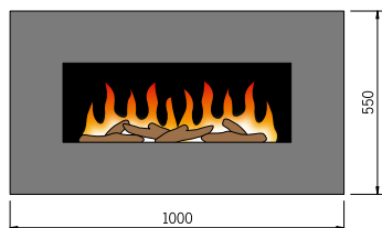
Singolo mit Blendrahmen
