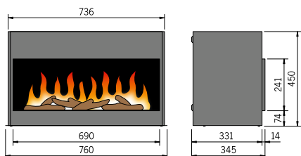
Singolo mit Blendrahmen
