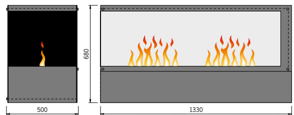
Inside-3S Slim mit 2 Brenner Medium
