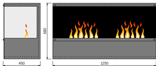
Inside-3S mit 2 Brenner Medium
