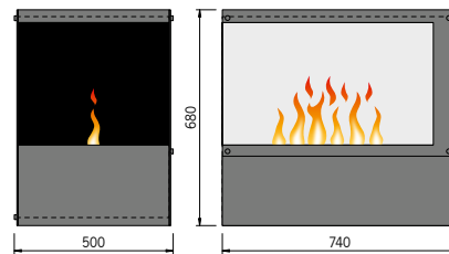
Inside-3S Slim mit 2 Brenner Medium
