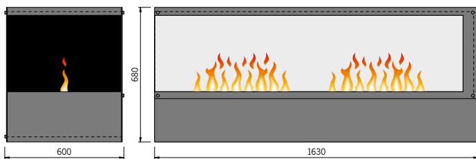
Inside-3S Slim mit 2 Brenner Large
