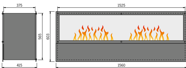
Inside-Tunnel mit 2 Brenner Large
