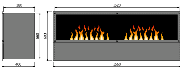
Inside-Front mit 2 Brenner Large
