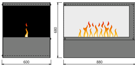
Inside-3S Slim mit 2 Brenner Large
