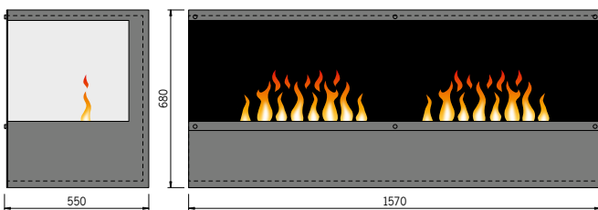
Inside-3S mit 2 Brenner Large
