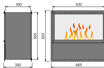
Inside-Tunnel mit 2 Brenner Medium
