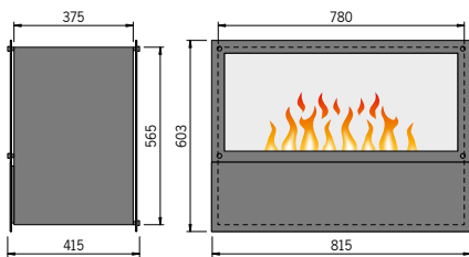
Inside-Tunnel mit 2 Brenner Large
