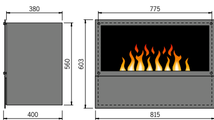
Inside-Front mit 1 Brenner Large
