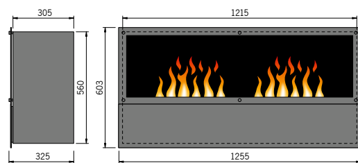
Inside-Front mit 2 Brenner Medium
