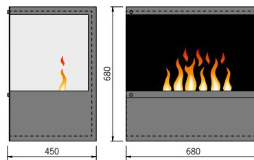
Inside-3S mit 2 Brenner Medium
