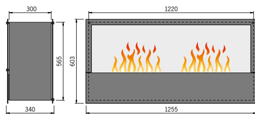
Inside-Tunnel mit 2 Brenner Medium
